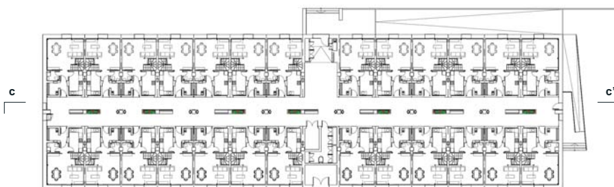
PLANTA BAJA
