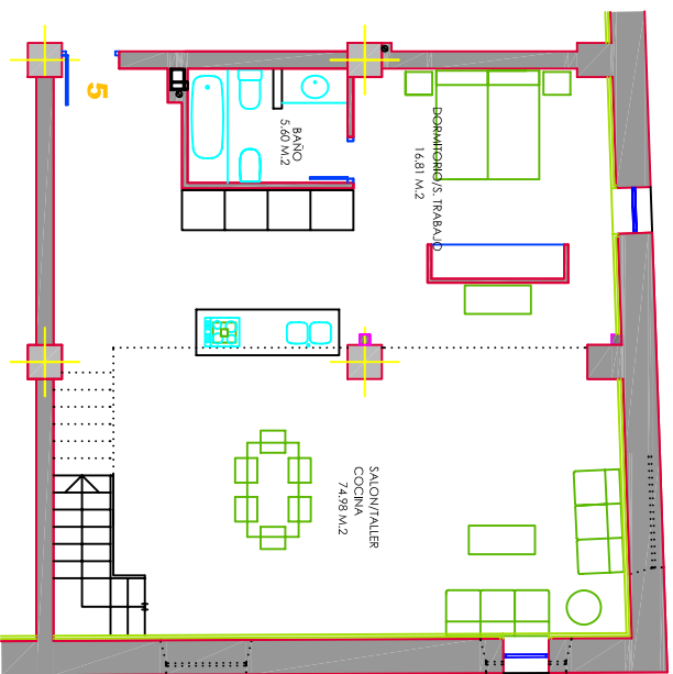
PLANTA BAJA
